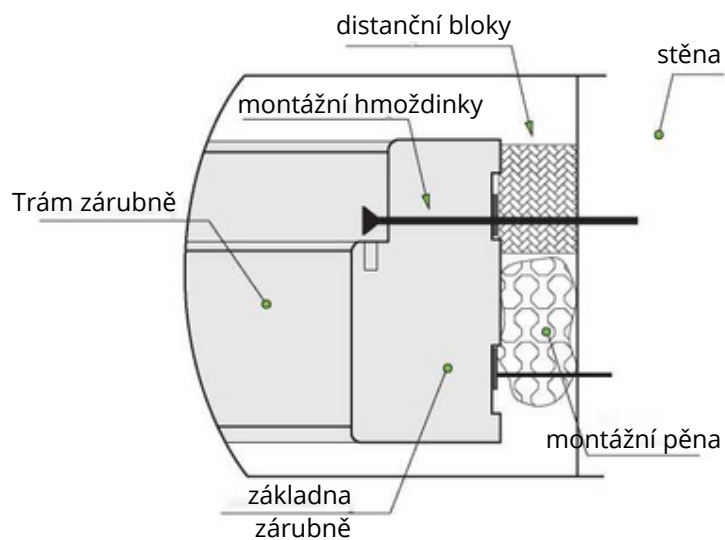
obr. 4 - Upevnění zárubně ke stěně (pohled zespodu)
