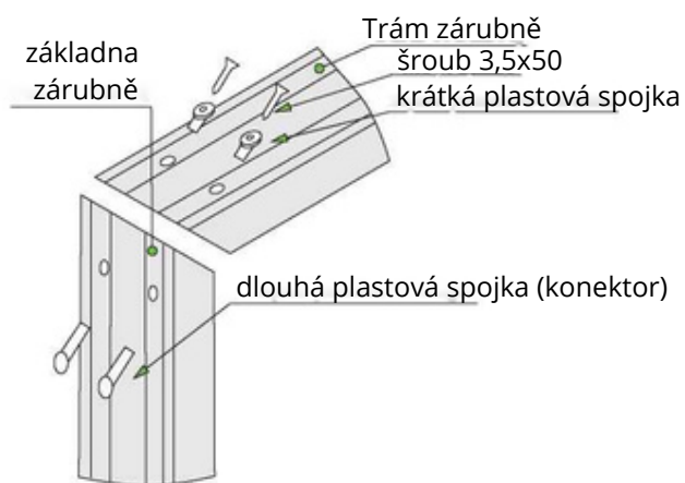
obr. 1 - Připojení zárubně pomocí spojek a šroubů
