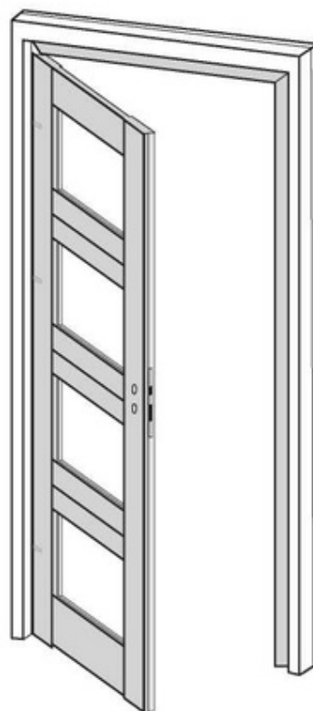
obr. 5 - Upevnění závěsů, osazení křídla v zárubni
