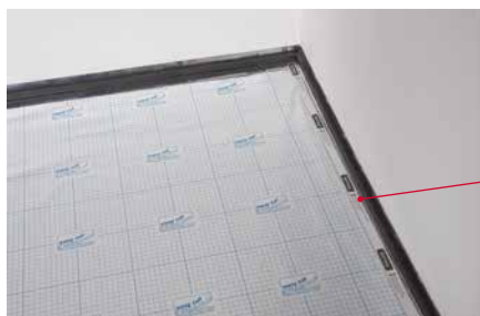
bariéra proti vlhkosti & těsnící páska
